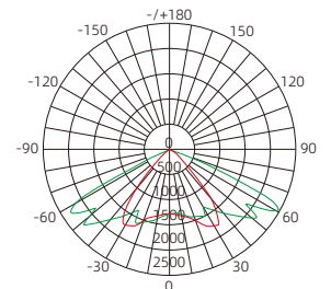
平均光束角 (50%) : 110.0度 The average beam angle (50%) : 110.0 Degree CZ0878/211 □-LED0060WWB
