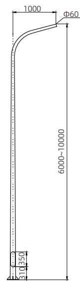
灯杆示意图
